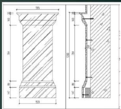
PHƯƠNG ÁN THI CÔNG CHÂN CỘT
