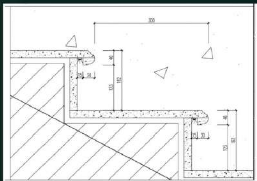
PHƯƠNG ÁN THI CÔNG BẬC THẤP
